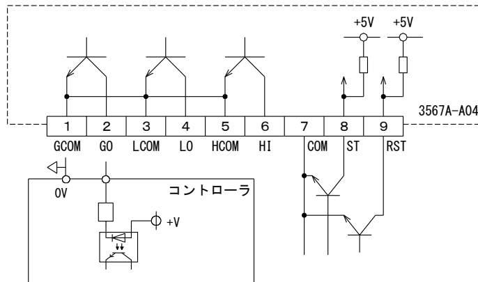
オープンコレクタ出力
