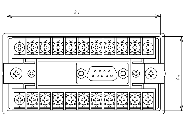
RS-232C出力付タイプ
