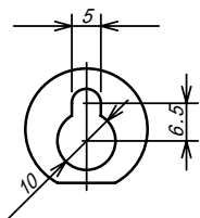
1 詳細図 (1:1)
