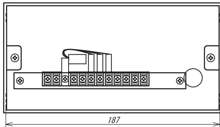
● 3155D-TCの場合
