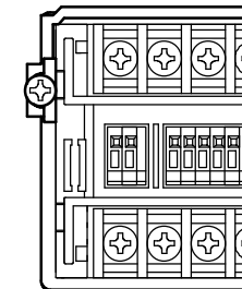
ANALOG+RS-232C, ANALOG+RS-485
