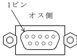
8528コネクタDサブ9ピン
