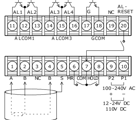
抵抗温度計
