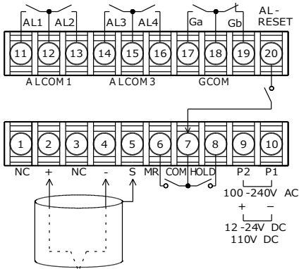
熱電温度計
