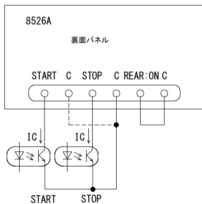
図13.1 リモートコントロール端子台接続例
