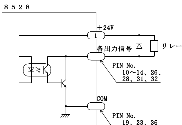
図13.2 リレードライブ接続例
