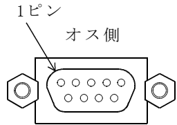
8528コネクタDサブ9ピン
