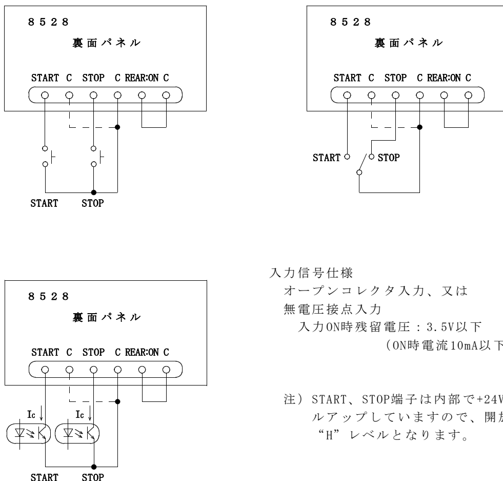
図12.1 リモートコントロール端子台接続例
