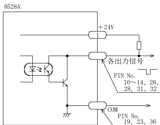
図13.3 信号レベルを得る例
