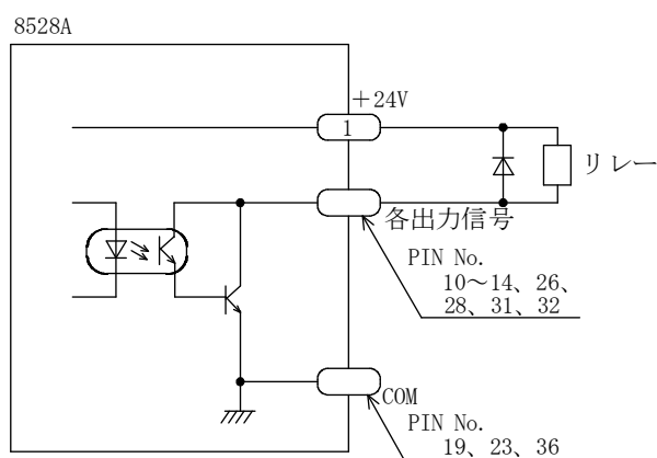
図13.2 リレードライブ接続例
